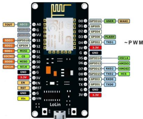
Figura 2 – Placa NodeMCU ESP8266_ pinagem. Fonte: AranaCorp.
